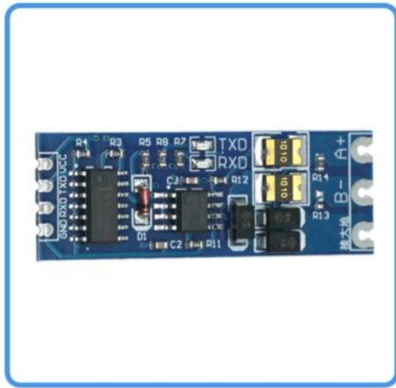
TTL-RS485 conversion module
