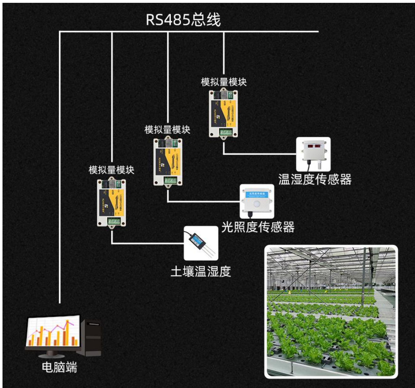
典型应用
