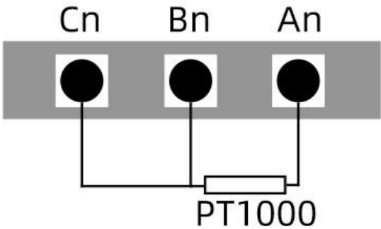
三线制接法
