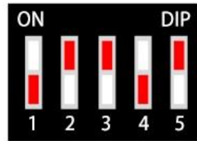
DC0~10V电压型
