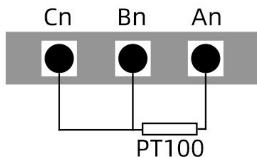
三线制接法
