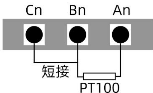
二线制接法
