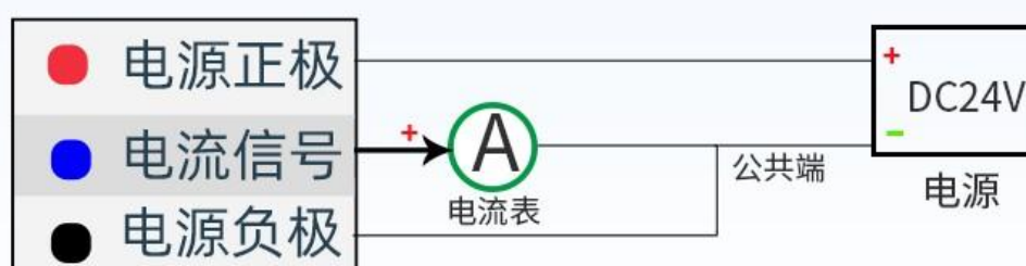
电流型接线示意图
