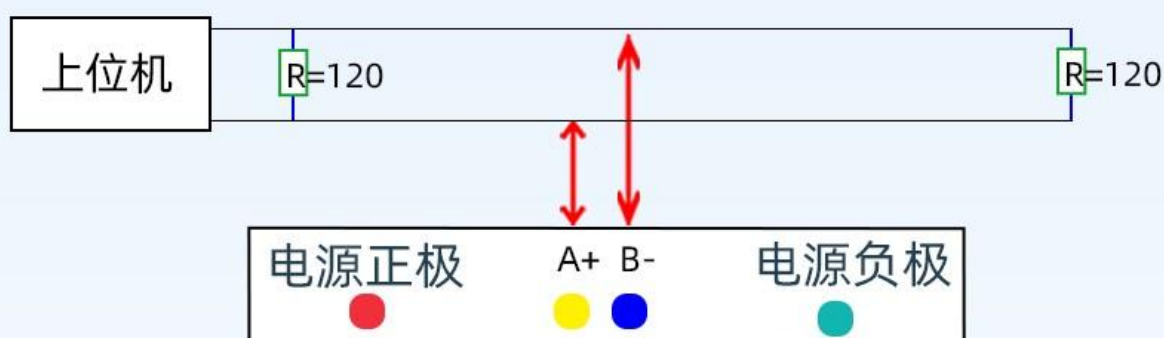
RS485接线示意图
