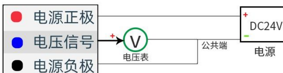
电压型接线示意图
