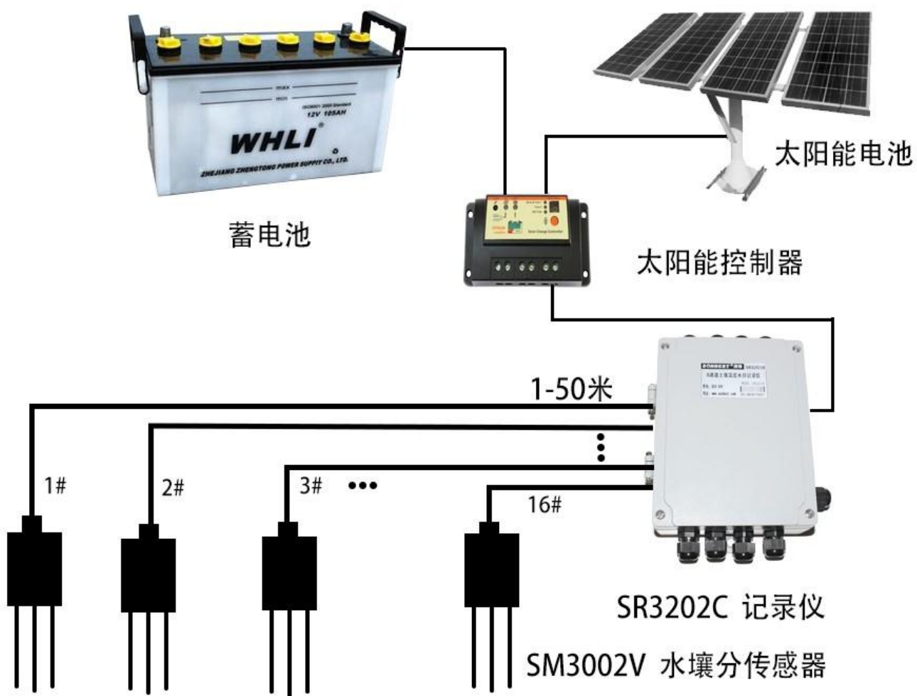
外部太阳能供电模式
