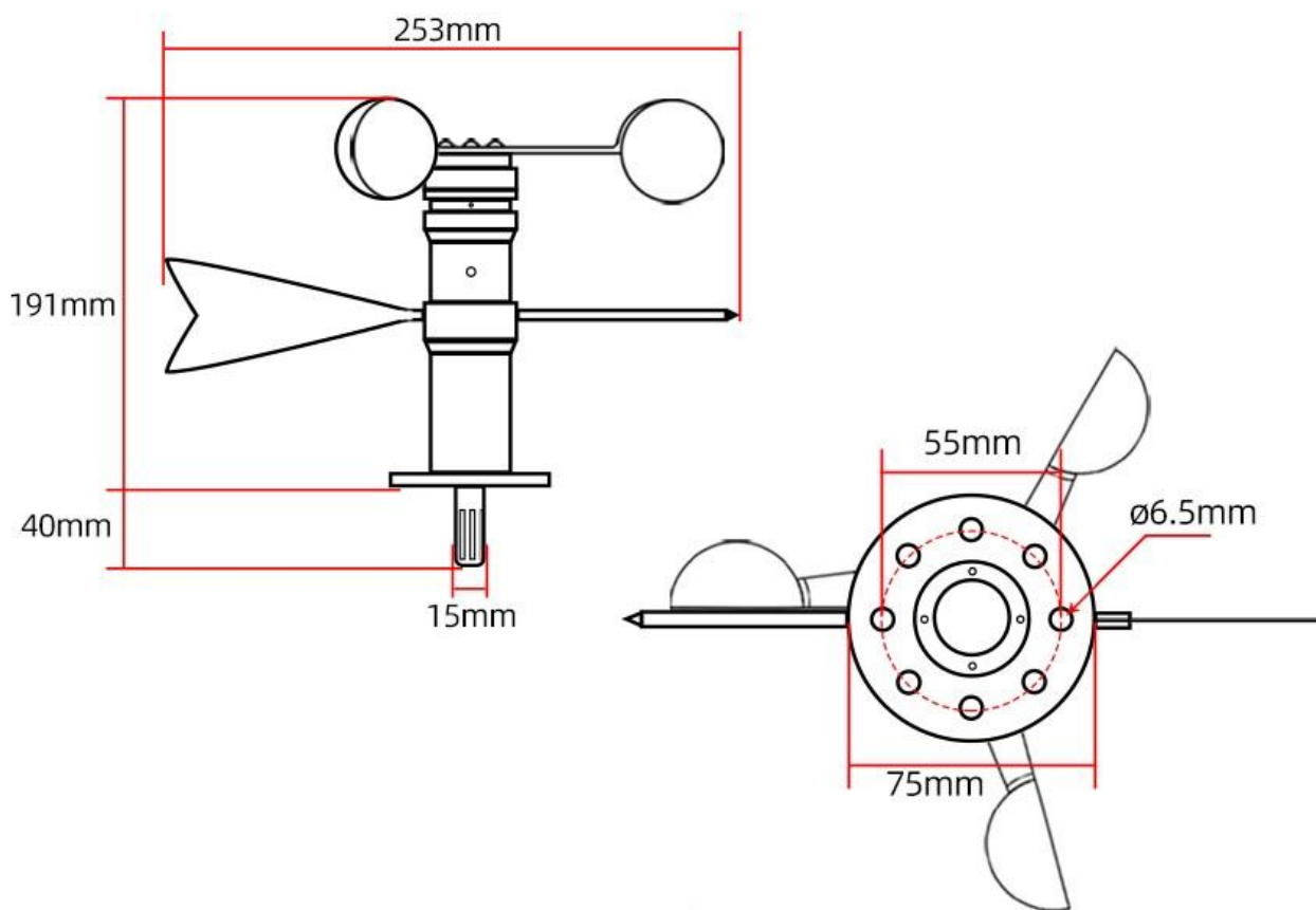
风速风向传感器尺寸图
