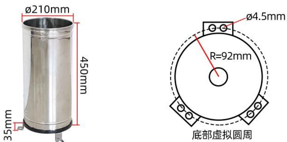
雨量传感器，蒸发量传感器尺寸图（两者尺寸相同）
