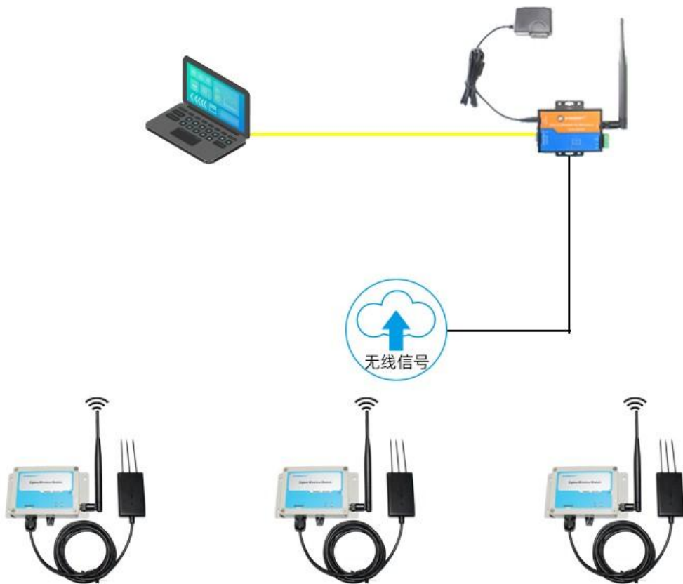
ZIGBEE模块支持多类型无线传感器
