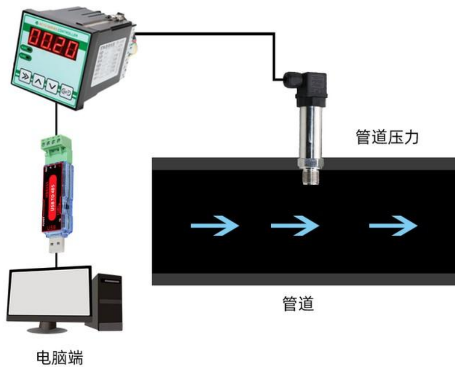
螺纹式安装方式
