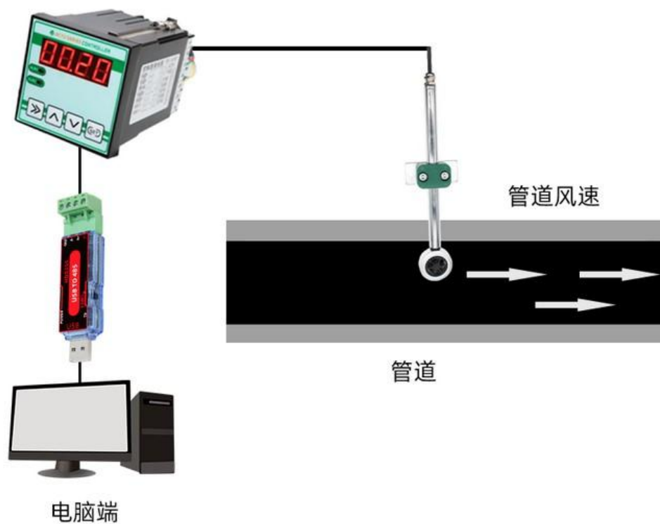
支架式安装方式
