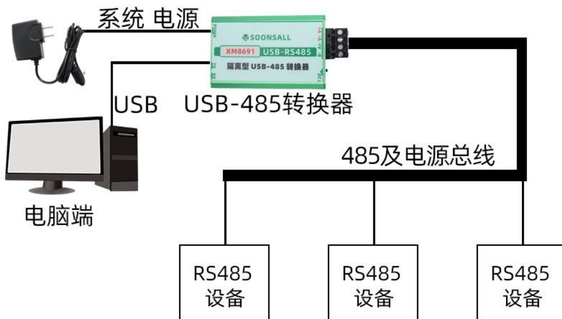
RS485系统共用电源方案
