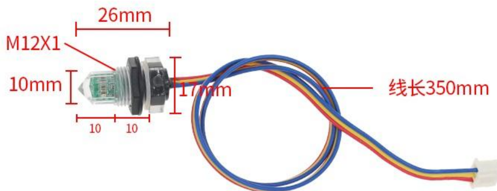
YN6938-1尺寸图
